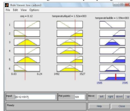
Gambar 7 Penalaran fuzzy
