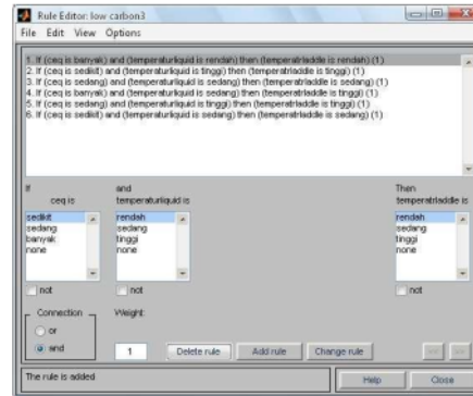
Gambar 6 Rule Pada Fuzzyfikasi Baja Low Carbon
